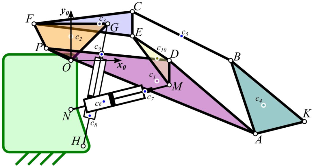
Rysunek 1. Schemat kinematyczny mechanizmu
